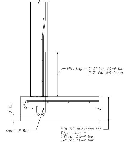
OPTIONAL HOOK DETAIL
